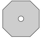
Låsbricka skala 1:1 Ca 20x20 mm Plastbit eller ca 2 mm tjock aluminiumplåt
